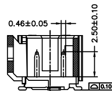
SEC: A-A
